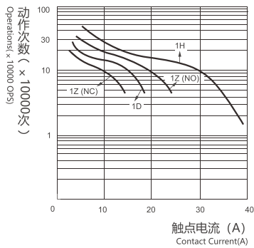
电耐久性曲线 ENDURANCE CURVE
